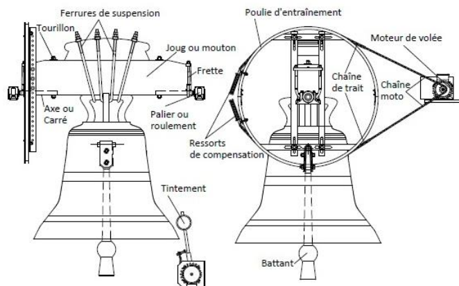
Eléments de sonnerie
